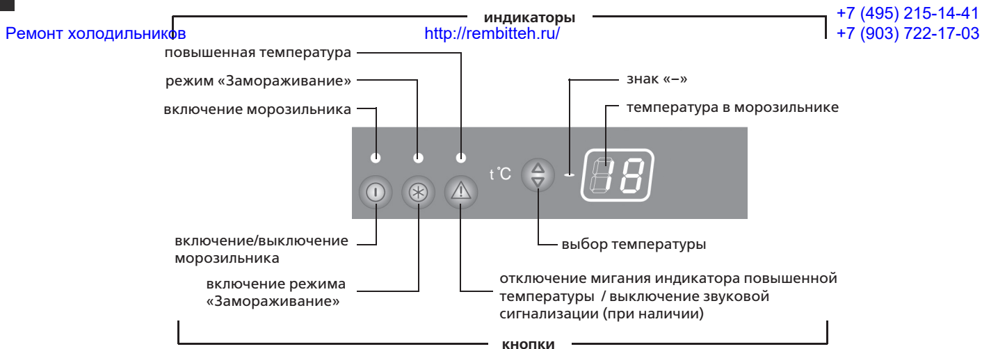
Рисунок 3 — Блок управления морозильника
