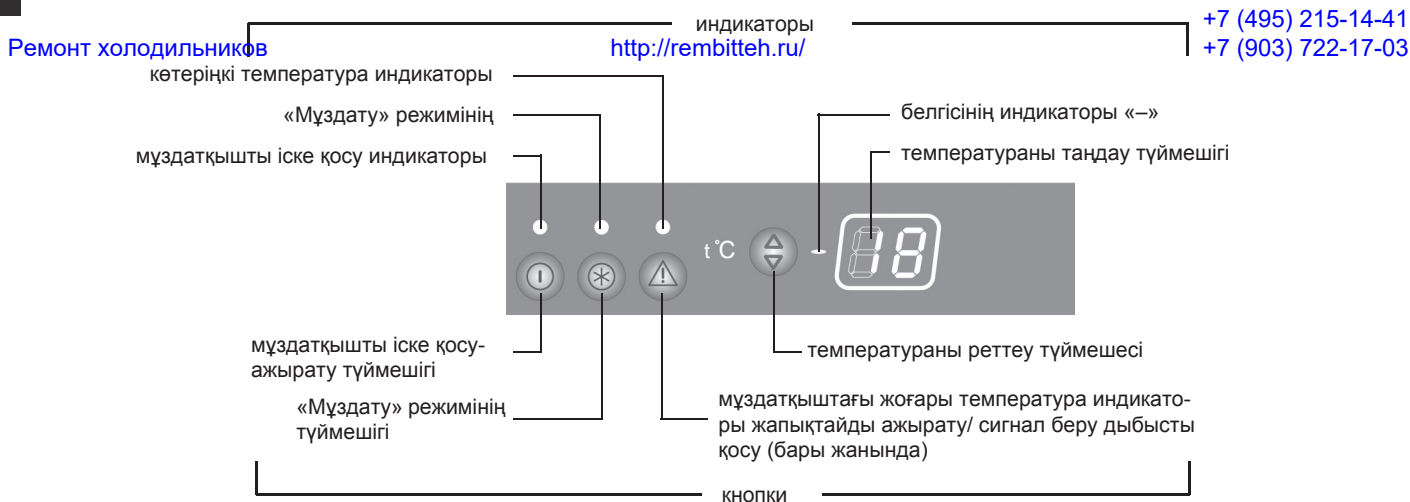
Сурет 3 – Басқару блогы
