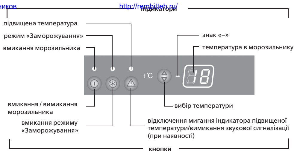
Рисунок 3 — Блок керування
