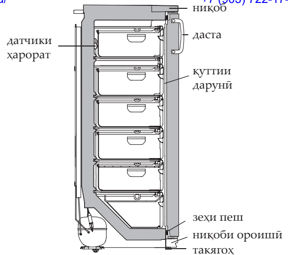
Расми 5 – Нақшаи сармодон
