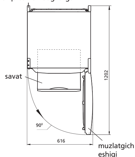
Rasmi 2 – Muzlatgich (yuqoridan ko'rinishi)
