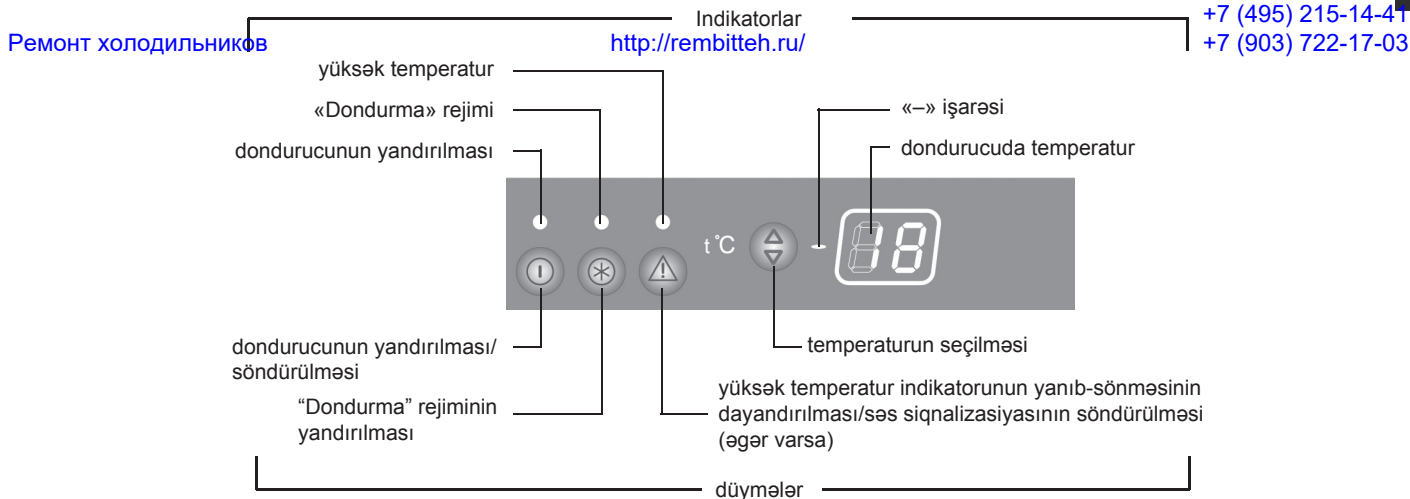
Şəkil 3 – İdarəetmə bloku
