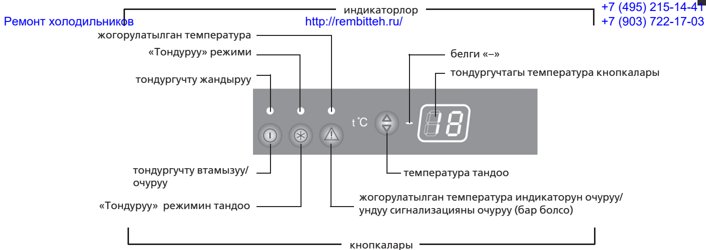
Сурот 3 — Башкаруу блогу
