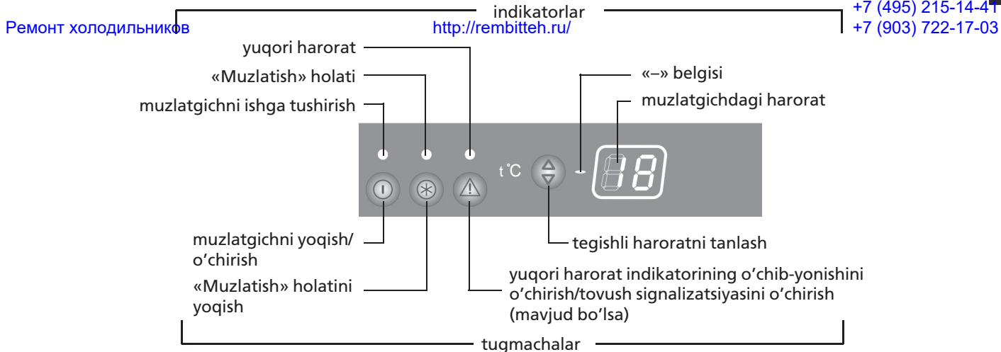
Rasmi 3 – Boshqaruv bloki
